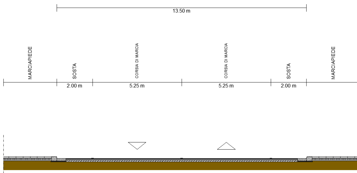
Figura 8.1: via Antonino Pio – tratto tra via Adriano e Traversa Antonino Pio, sezione trasversale esistente.
