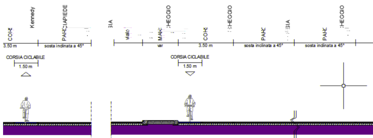
Figura 14.2: viale John Fitzgerald Kennedy – primo tratto: sezione trasversale di progetto.
